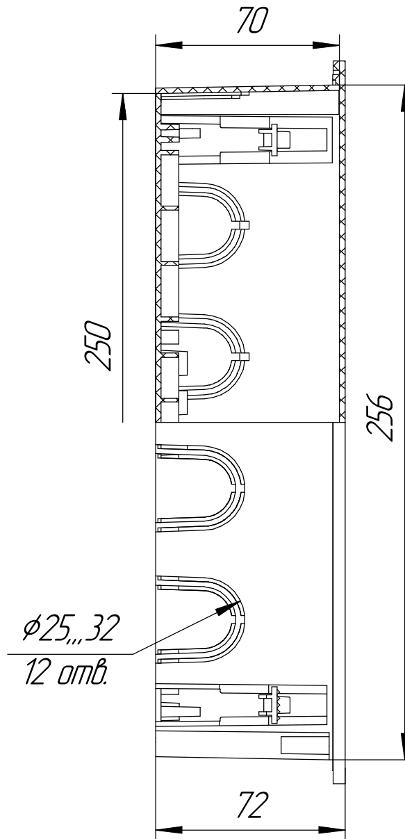
Коробка распределительная 80-0980 для с/п безгалогенная (HF) 256x171x70
