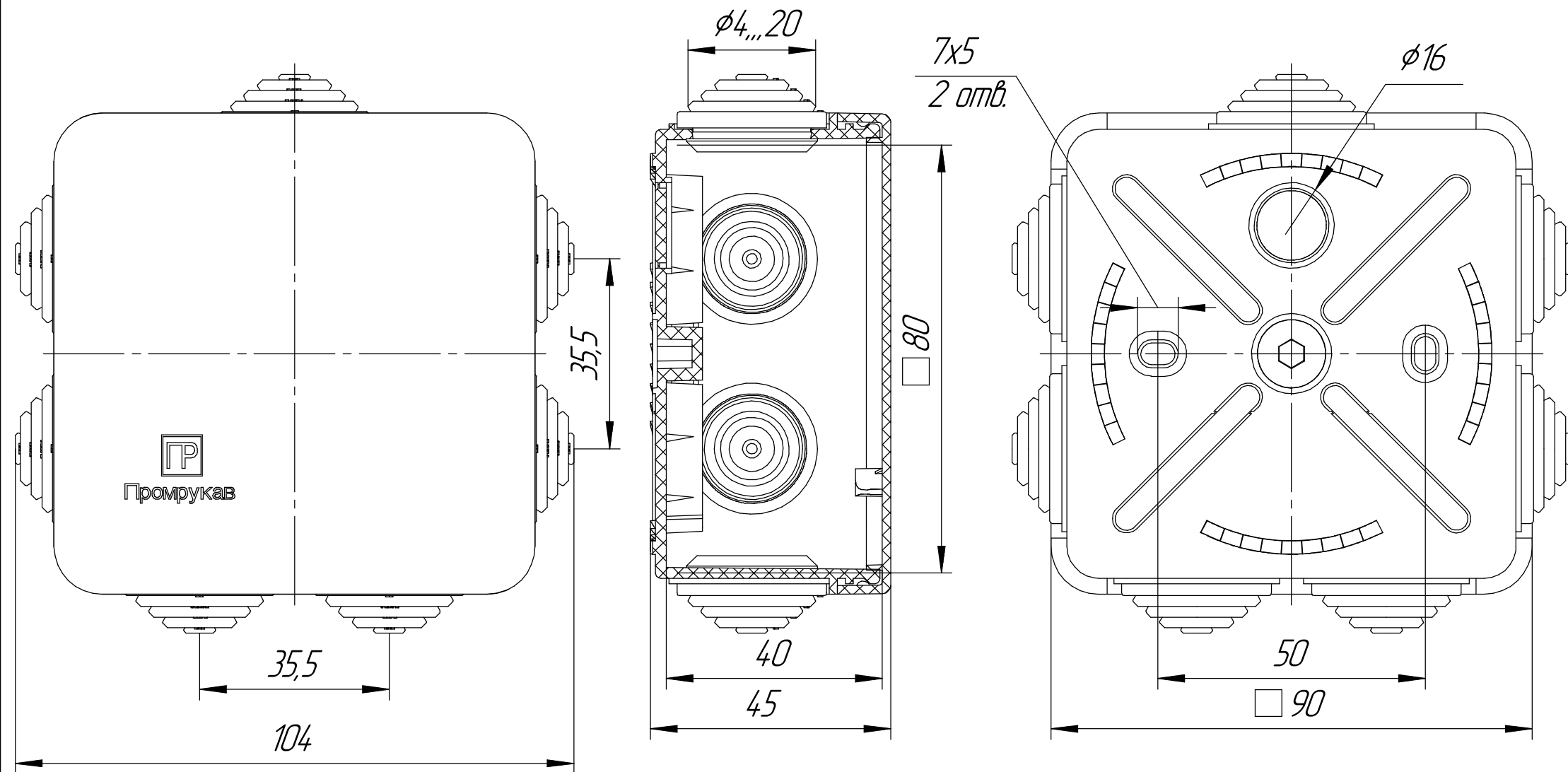
Коробка распределительная 40-0210 для о/п безгалогенная (HF) 80x80x40
